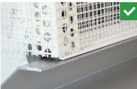
Abb. 48 mit Putzabschlussprofil mit integriertem Fugendichtungsband sowie stirnseitigem Anschluss mit Fugendichtungsband BG 1
